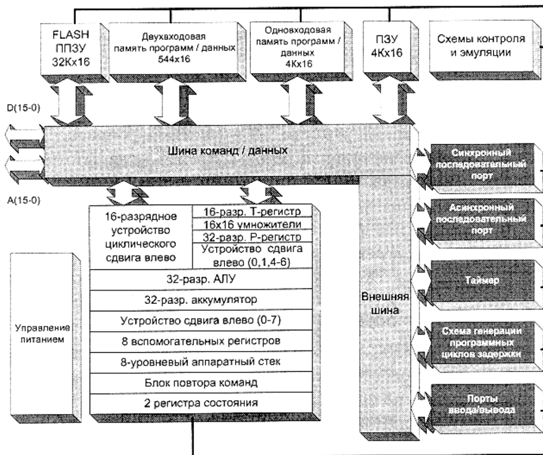
Рис. 4.1. Структура ПЦОС TMS320C2xx
