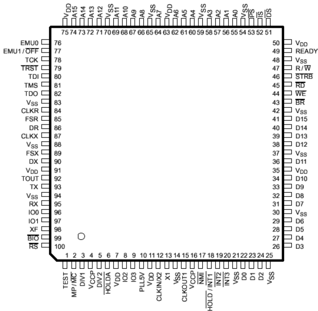
Рис. П.3. Расположение выводов ПЦОС TMS320F206 (вид сверху)
