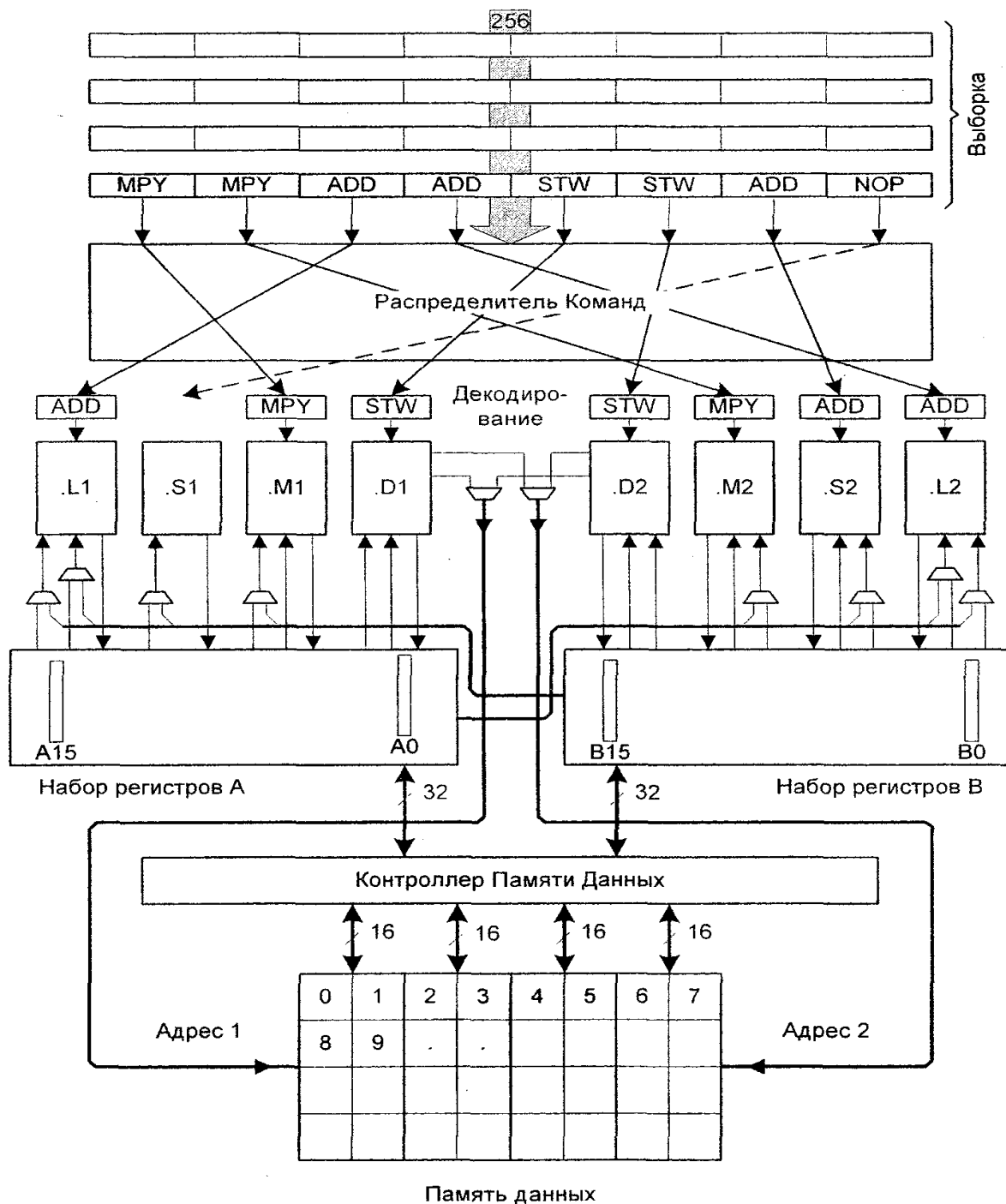
Рис. 6.2. Архитектура Velocity
